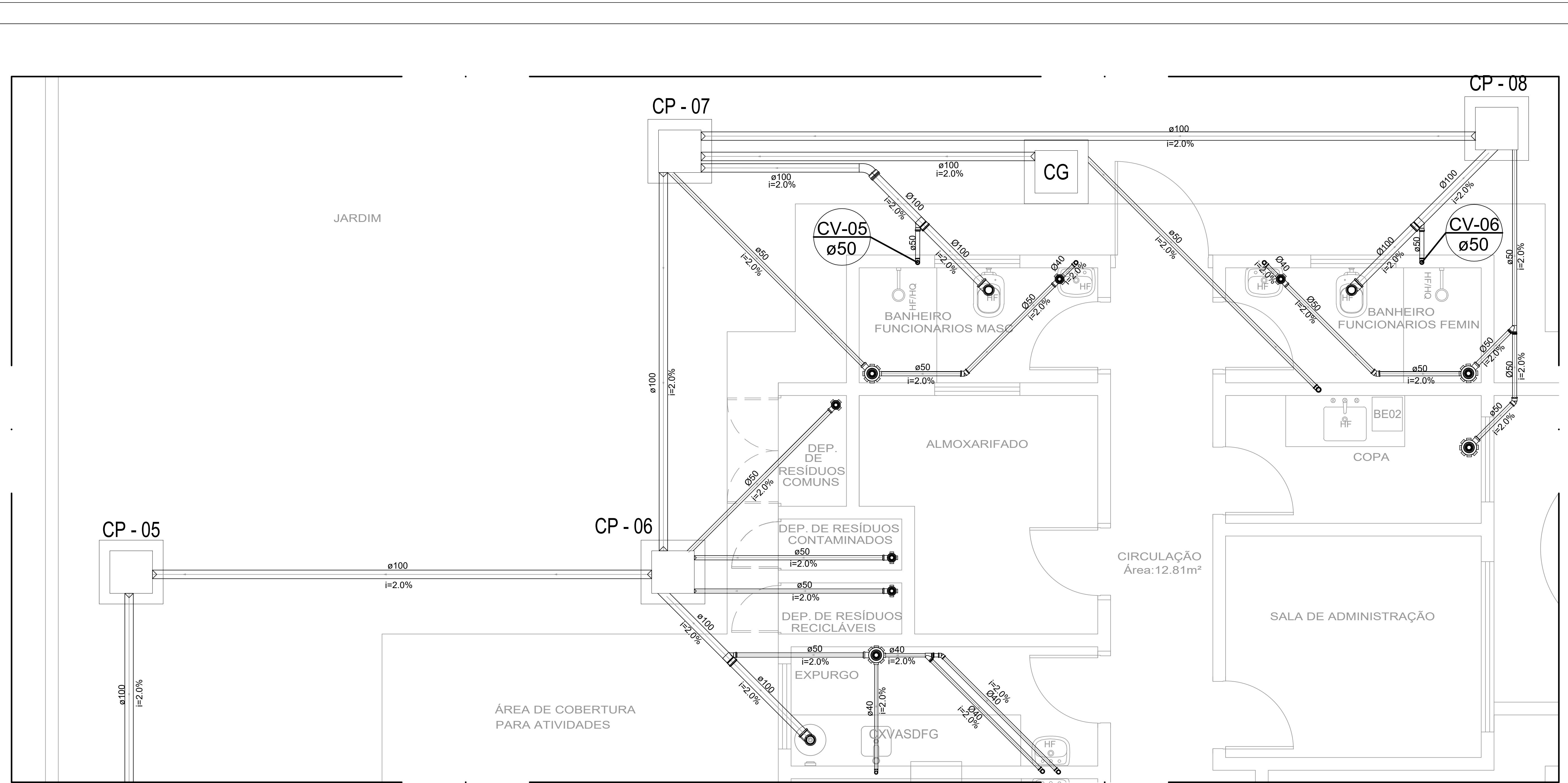
DETALHE DE ESGOTAMENTO SANITÁRIO - 04 ESCALA 1:25
